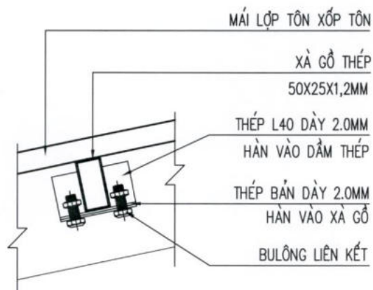
CHI TIẾT LIÊN KẾT XÀ GỖ VỚI DẦM THÉP (TỶ LỆ : 1/5)
