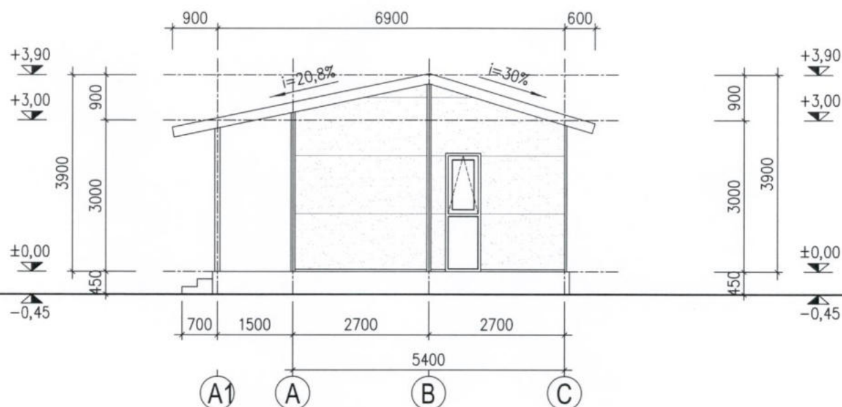
MẶT ĐỨNG BÊN (TỶ LỆ : 1/100)
