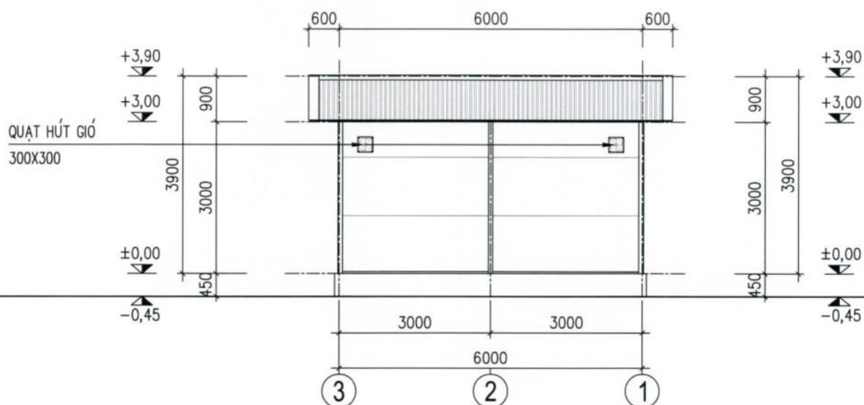
MẶT ĐÚNG SAU (TỶ LỆ : 1/100)
