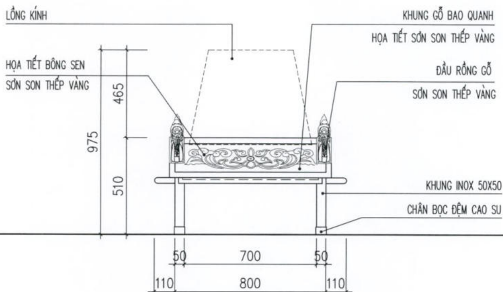
MẶT CHÍNH GIÁ KHIÊNG
