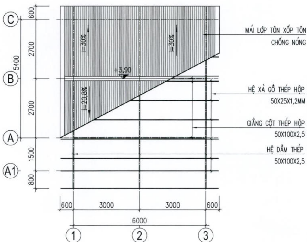
MẶT BẰNG MÁI (TỶ LỆ : 1/100)
