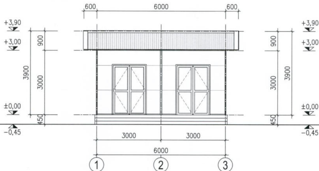
MẶT ĐÚNG CHÍNH (TỶ LỆ : 1/100)
