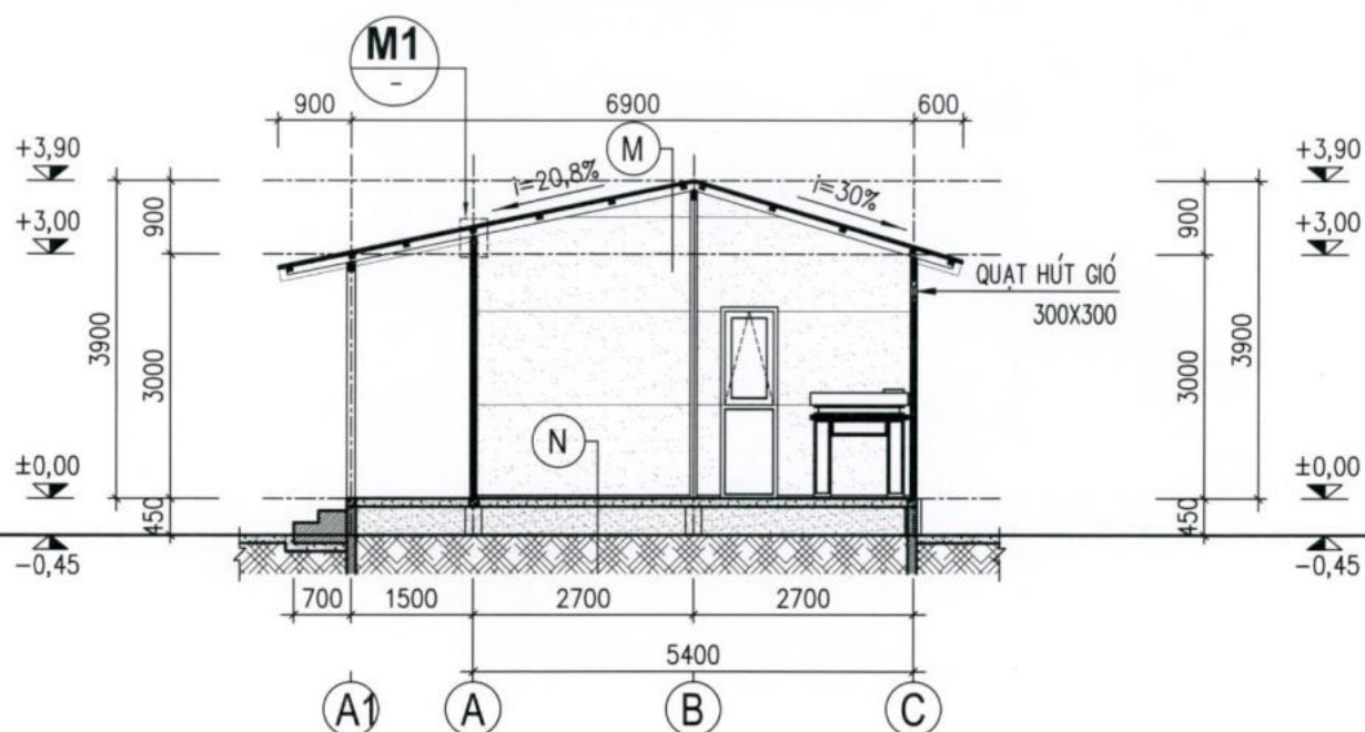
MẶT CẮT 1-1 (TỶ LỆ : 1/100)
