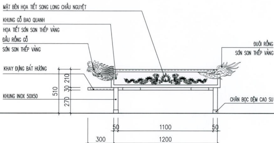
MẶT BÊN GIÁ KHIÊNG
