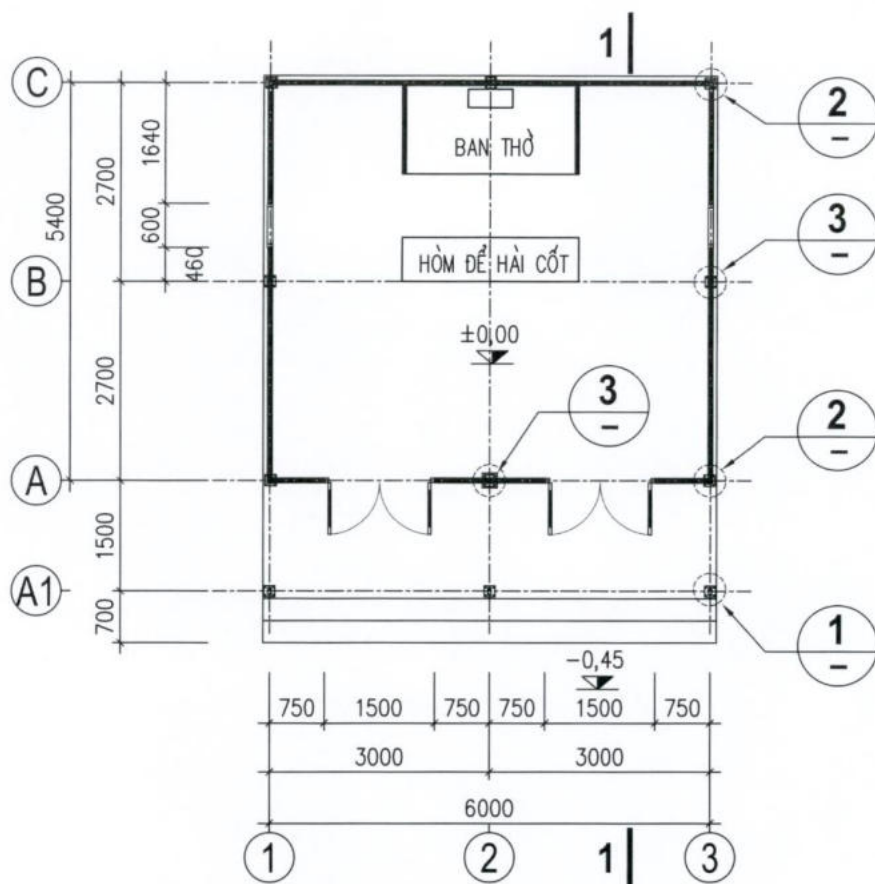
MẶT BẰNG TẦNG 1 (TỶ LỆ : 1/100)
