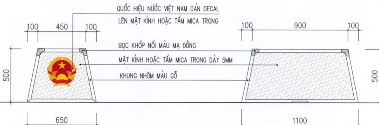
MẶT CHÍNH LỒNG KÍNH
