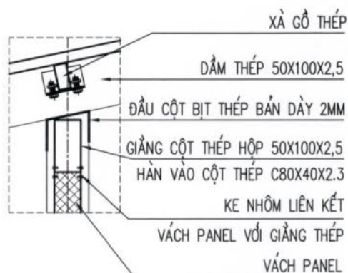
CHI TIẾT (M1) TỶ LỆ : 1/10
