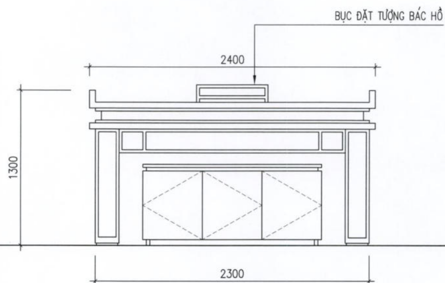
MẶT ĐỨNG CHÍNH
